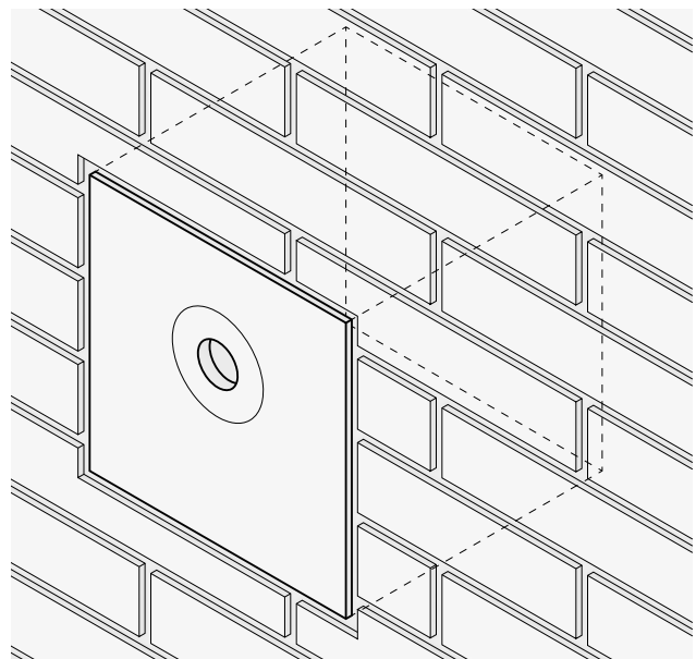
In Fassade eingebauter Nistkasten für Haussperlinge
